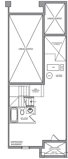
BASEMENT ELEVATION A1 & A2
