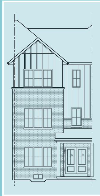
ELEVATION B2
